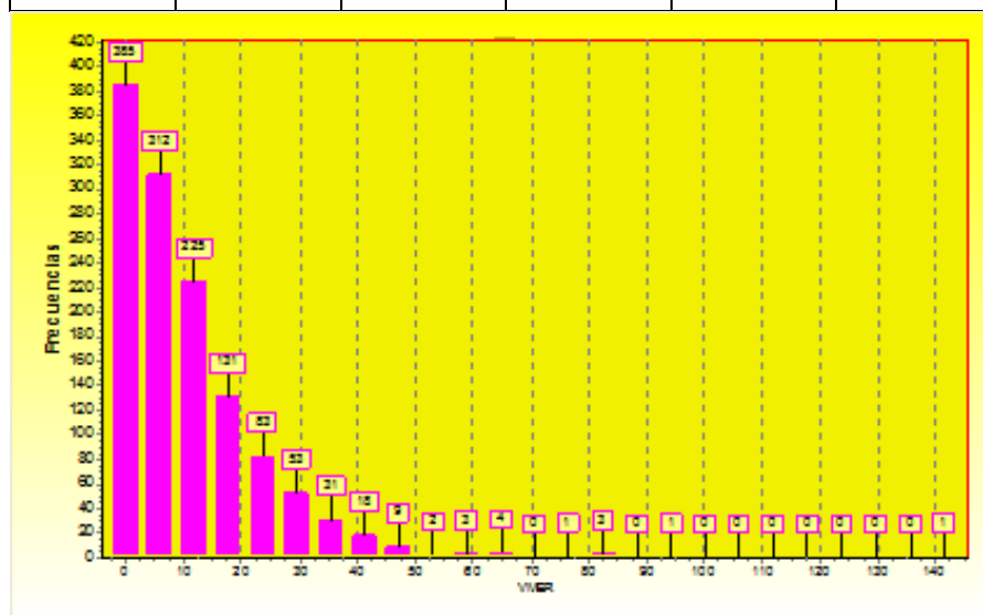
Figura 2. Modelación del comportamiento dentro de la frontera de R3, según MPL, estadística básica y distribución de frecuencias de VMER para la variable N_i .
