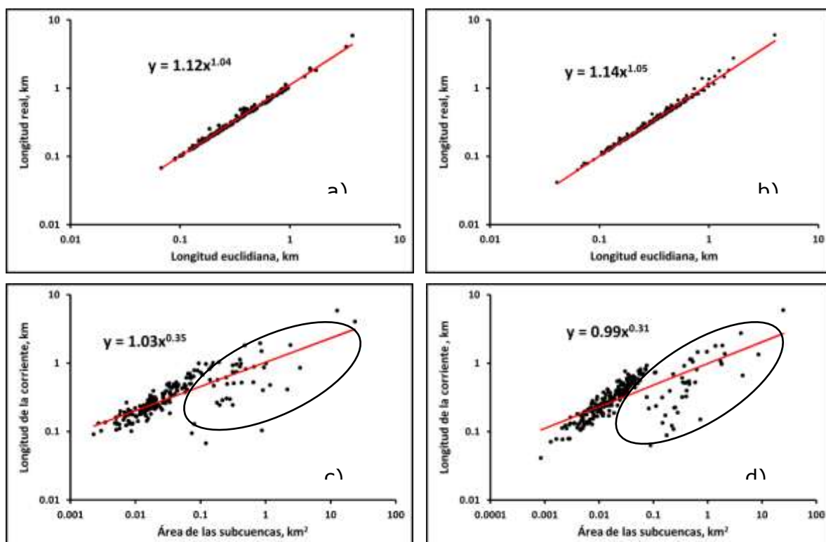
Figura 3. Determinación de la dimensión fractal promedio de la corriente para los ríos San Cristóbal y Santa Cruz a partir de las pendientes de las rectas ajustadas. a) y b) según Takayasu (1990); c) y d) según Mandelbrot (1983). Las elipses encierran los ríos que se alejan de la nube principal, mayormente de orden dos en adelante.
