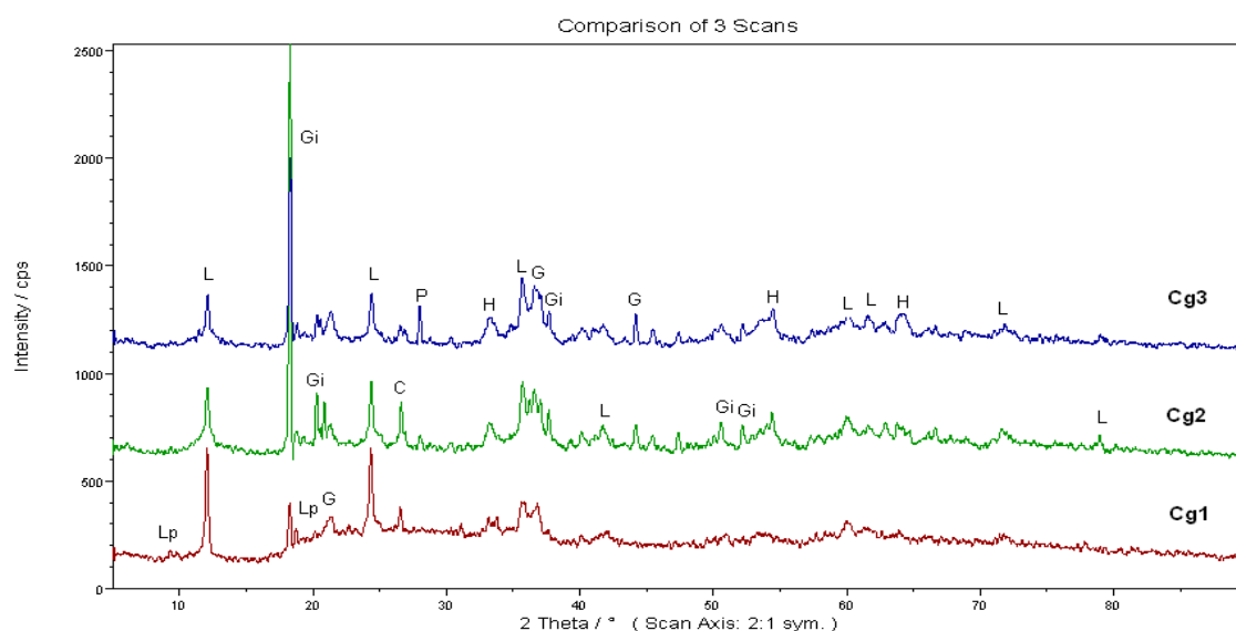
Figura 5. Difractograma de rayos -X de las fracciones granulométricas (-10+8mm); (-8+4 mm); (-4+2 mm). G: Goethita, Gi: Gibbsita, H: Hematita, L: Lizardita, C: Cuarzo
