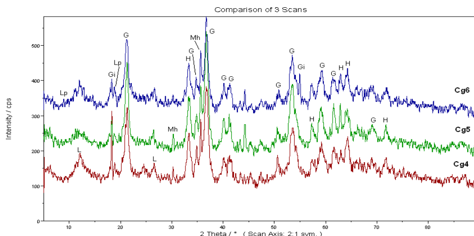
Figura 6. Difractograma de rayos -X de las fracciones granulométricas (-2+1 mm); (-1+0,4 mm); (-0,4+0,2 mm). G: Goethita, Gi: Gibbsita, H: Hematita, L: Lizardita, Mh: maghemita, Lp: Litioforita.
