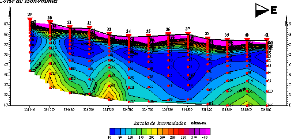
Figura 12. Corte de resistividad aparente \rho_a con curvas de tipo "H", meseta de Cajalbana, Pinar del Río, perfil 1.
