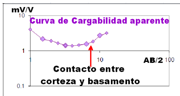
Figura 10. Puntos característicos de la curva de tipo "H" de cargabilidad aparente C_a , yacimiento Pinares de Mayarí Oeste, bloque I19115, pozo 03.
