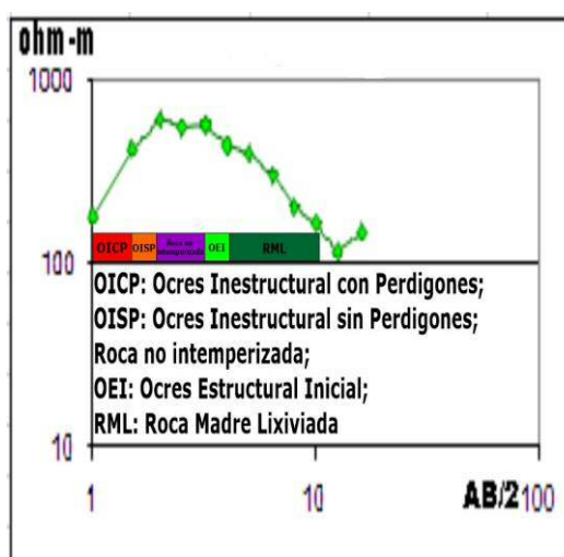
Figura 8. Curva de resistividad aparente pa de tipo "K" con litología asociada, yacimiento Yagrumaje Norte, bloque 0758, pozo 05.
