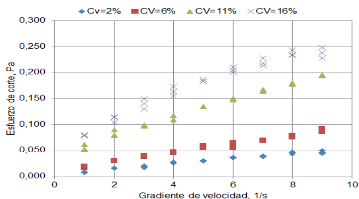
Fig. 2. Curva de flujo para las distintas concentraciones de sólidos en volumen
