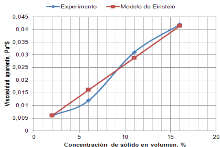
Fig. 3. Gráfico de comparación de la viscosidad aparente obtenida y la predicha
