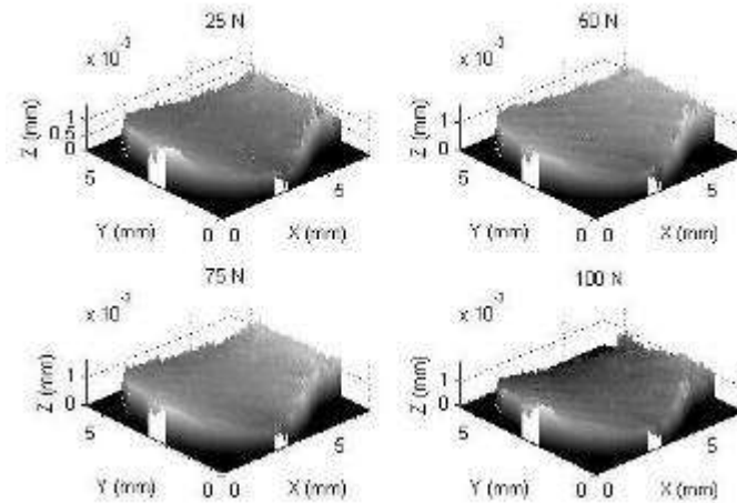
Fig. 10. Imágenes de deformación superficial para las fuerzas aplicadas de 25 N-100 N (dientes A3-MOD-Amalgama)
