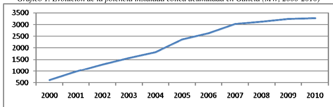
Gráfico 1. Evolución de la potencia instalada eólica acumulada en Galicia (MW, 2000-2010) 4
