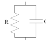
Figura 12. Modelo eléctrico del aterrizamiento del electrodo sobre la muestra de suelo
