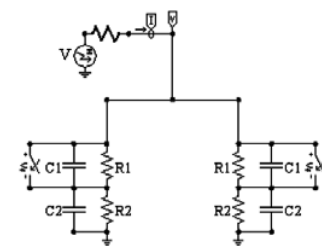
Figura 20. Modelo de la suela del zapato e impedancia de aterrizamiento analizado en EMT/ATP. Para este caso específico, se simularon dos caminos de corriente diferentes.
