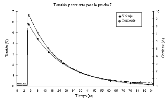
Figura 9. Señales de tensión y corriente en función del tiempo para la prueba 7.
