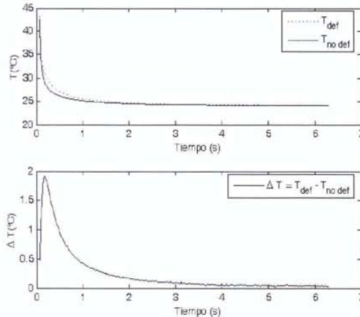
Gráfica 2. Curvas de temperatura y contraste térmico entre un área defectuosa y un área no defectuosa
