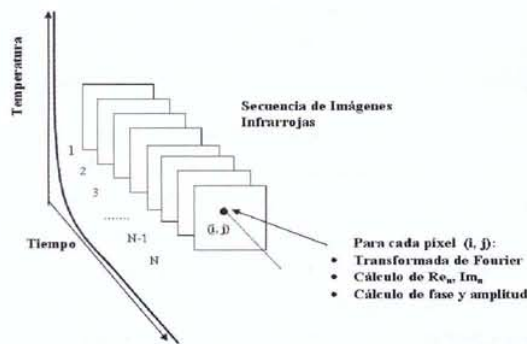
Figura 2. Termografía de fase pulsada (PPT)
