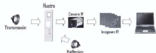
Figura 1. Configuración experimental para la termografía activa pulsada
