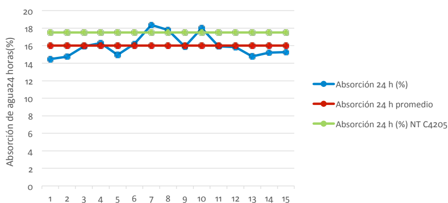
Figura 8. Absorción de agua 24 horas
