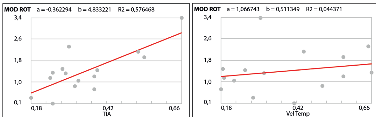
Figura 11. Regresión lineal múltiple TIA, velocidad con respecto al módulo de rotura
