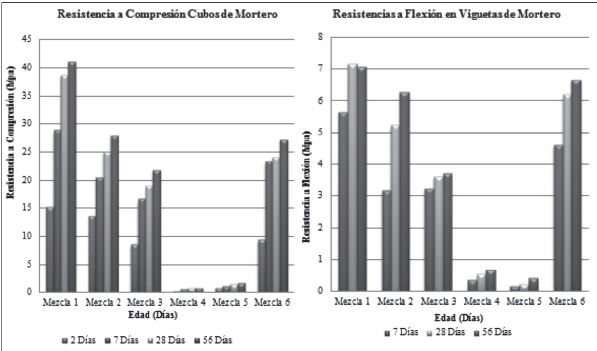
Figura 1. Resistencia a compresión y a flexión de probetas de mortero en las distintas edades evaluadas
