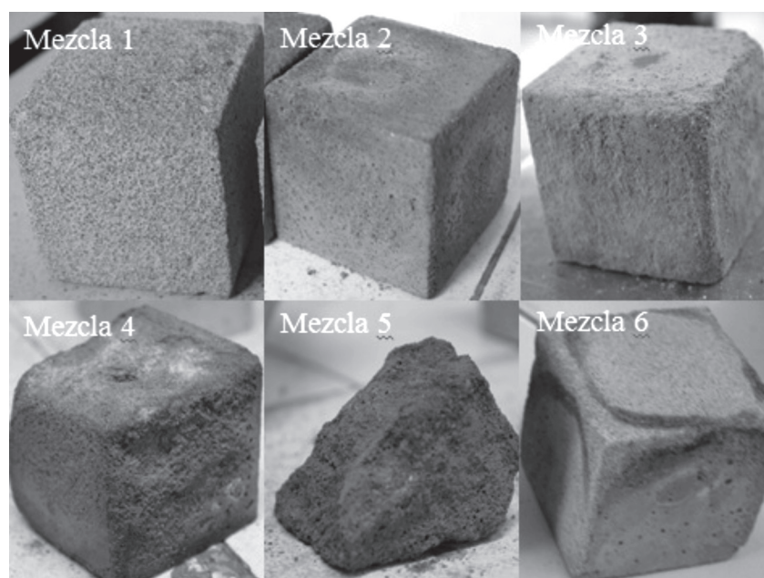
Figura 6. Pérdida de masa de cubosexpuestos a ataque de ácidos (a) mezcla 1; (b) mezcla 2; (c) mezcla 3; (d) mezcla 4; (e) mezcla 5, y (f) mezcla 6
