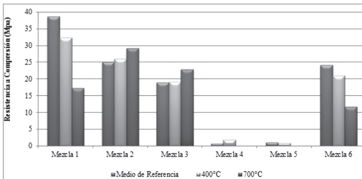
Figura 2. Resistencia a compresión, comparación con las probetas no expuestas a altas temperaturas
