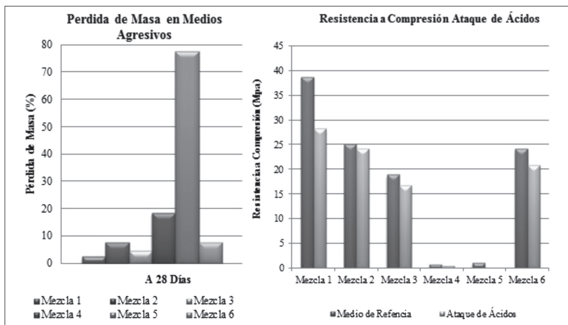
Figura 5. Pérdida de masa por exposición ante ácido sulfúrico y resistencia a compresión ante exposición de ácido sulfúrico vs. medio de referencia
