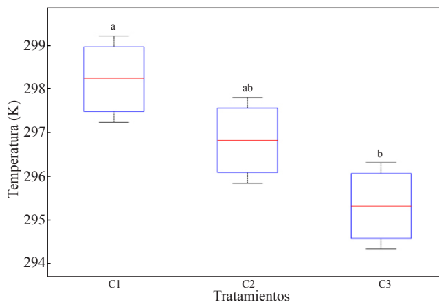
Figura 9. Comparación de medias de la temperatura interior promedio producida en el invernadero bajo tres configuraciones del sistema mecánico de ventilación. C1, C2, y C3 se refieren a la configuración 1, configuración 2 y configuración 3, respectivamente.
