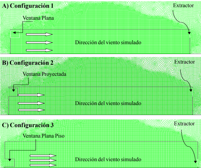
Figura 2. Escenarios de simulación y características de la malla. A) ventana plana y extractor en la cumbrera; B) ventana proyectada al interior y extractor en la cumbrera; y C) ventana proyectada al interior y extractor a nivel del suelo.
