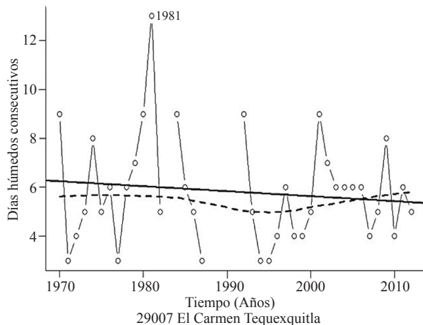
Figura 3. Variabilidad anual de los días húmedos consecutivos.
