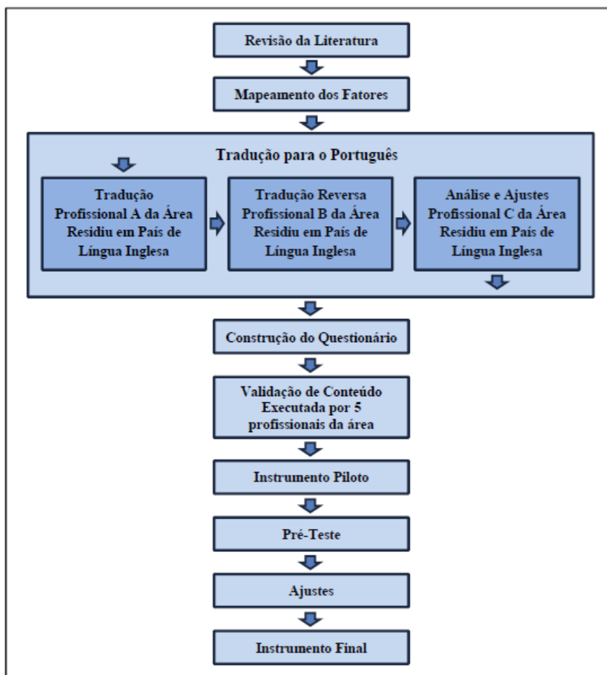
Figura 2: Percurso Metodológico
