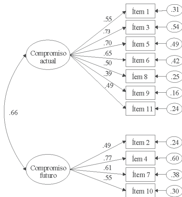
FIGURA 1: Análisis factorial confirmatorio del modelo de dos factores de la Escala de Grado de Compromiso hacia el Deporte de Orlick (2004). Las elipses representan los factores o dimensiones de la escala y los rectángulos muestran los diferentes ítems. Todos los pesos de regresión están estandarizados y son estadísticamente significativos ( p < .05 ). Las varianzas del error están representadas por los círculos pequeños.
