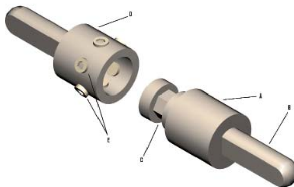
Figura 1. Desenho esquemático da prótese modular diafisária com suas respectivas estruturas. A- Segmento macho da prótese. B- Haste intramedular. C- Eixo central sextavado. D- Segmento fêmea da prótese. E- Parafusos sextavados.
