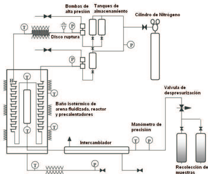
Figura 2. Esquema tecnológico de la unidad continua construida
