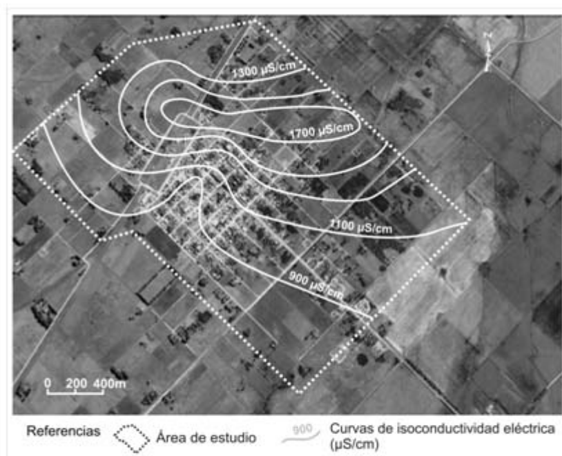
Figura 4. Mapa de isoconductividad eléctrica en María Ignacia (09/2012).
