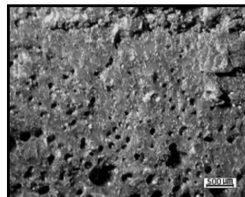
Fig. 9: Micrografía de PEZI4012 – 10X
