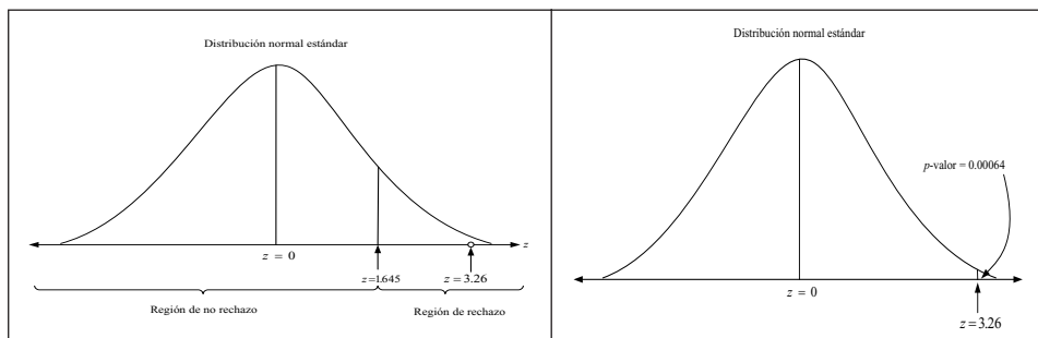
Figura 2. Distribución muestral de un estadístico de prueba con regiones de rechazo y aceptación y valor de p.
