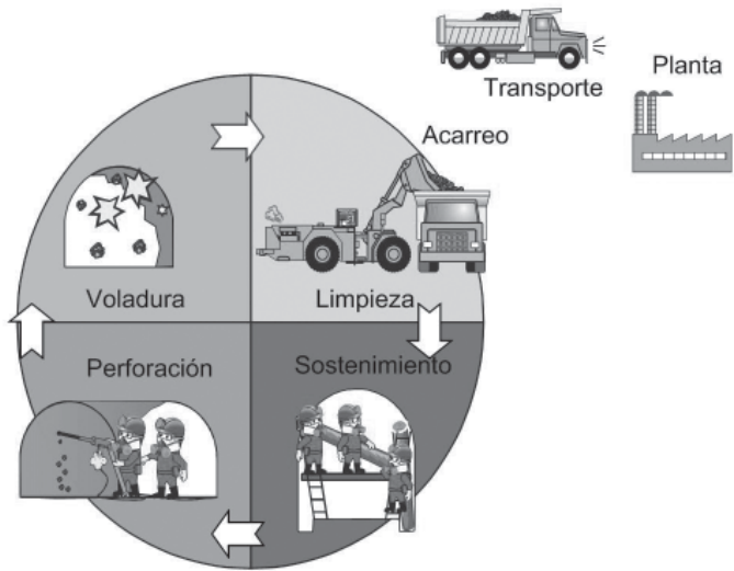
Figura 2 Proceso productivo del ciclo de minado
