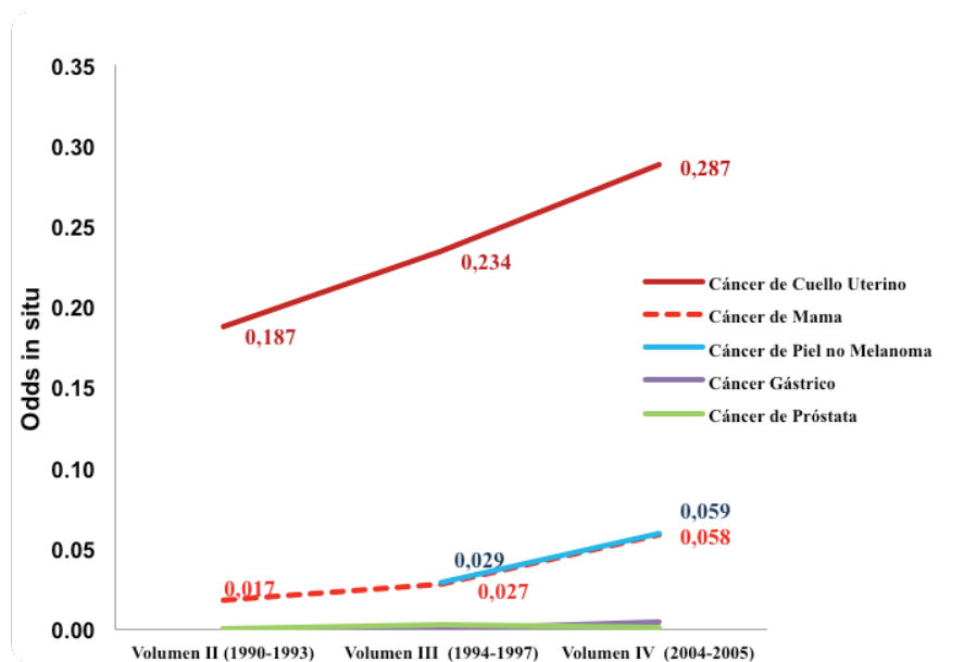
Gráfico 1. Odds in situ para cinco tipos de cáncer.
