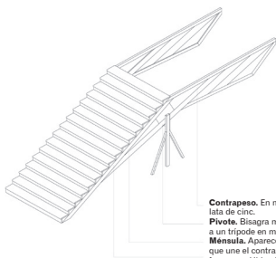
Figura 17. Modelo tipología bisagra
