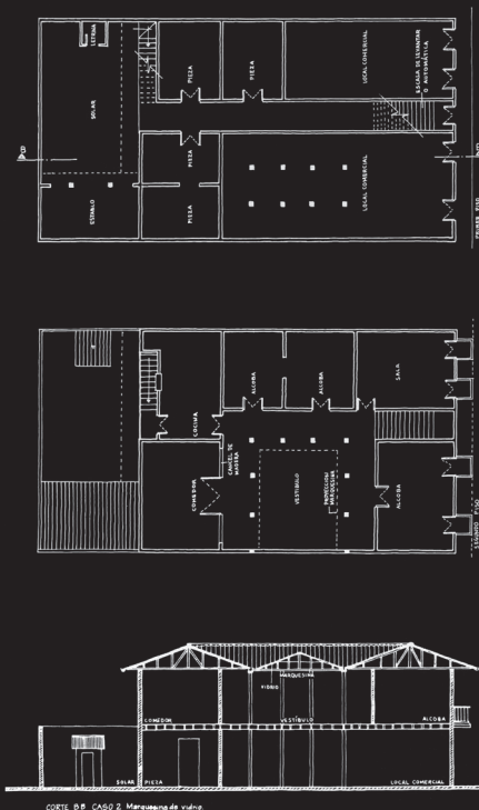
Figura 8. Vivienda de vestíbulo: plantas y cortes. En estos esquemas se observa cómo la vivienda fue sufriendo modificaciones por los cambios sociales y económicos. Aparece el vestíbulo, locales comerciales, cuartos o piezas de arriendo y la escalera pivotante en la parte del zaguán. Fuente: tomados de Robledo Castillo, La ciudad en la colonización antioqueña , 203-204
