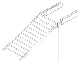
Figura 15. Modelo tipología barra
