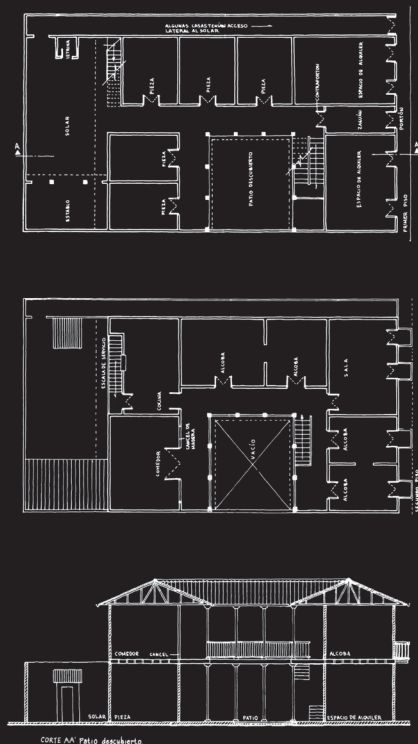
Figura 7. Vivienda de patio central: plantas y corte. Esquema básico de la vivienda antes de los cambios sociales y económicos; una vivienda de arraigo rural. Fuente: tomados de Robledo Castillo, La ciudad en la colonización antioqueña , 199
