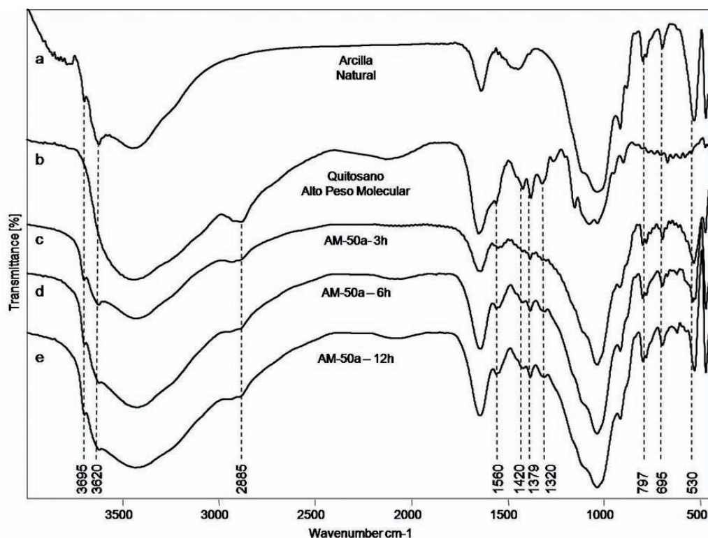
Figura 5. Espectros IR de (a) Arcilla natural, (b) Quitosano de alto peso molecular, y arcillas modificadas con este quitosano al 50% p/p con distintos tiempos de procesamiento: (c) 3 horas, (d) 6 horas, y (e) 12 horas.
