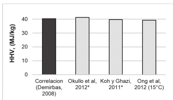
Figura 9. Poder calorífico superior del biodiésel de J. curcas . * Okullo et al. , 2012 y Koh y Ghazi, 2011 y reportan rangos, con valores mínimos de 41,2 MJ/kg y 39,23 MJ/kg, respectivamente.
