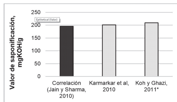
Figura 4. Valor de saponificación del aceite de J. curcas *Koh y Ghazi, 2011 reporta un rango, con valor mínimo de 102,9 mgKOH/g.
