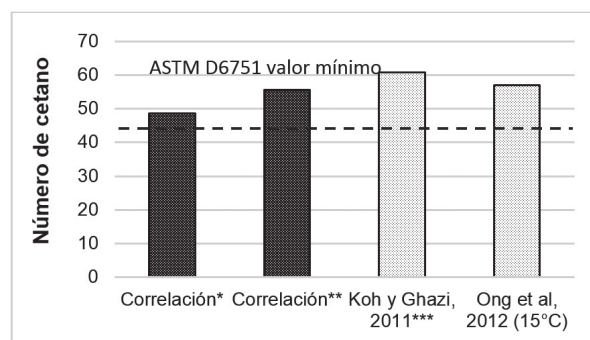
Figura 10. Número de cetano del biodiésel de J. curcas . *Wang et al. , 2012, **Ramírez-Verduzco et al. , 2012, ***Koh y Ghazi, 2011 reporta un rango, con valor mínimo de 60,74.
