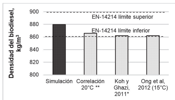
Figura 8. Densidad del biodiesel de J. curcas . *Koh y Ghazi, 2011 reporta un rango, con valor mínimo de 858kg/m 3 , **Ramírez-Verduzco et al. , 2011.
