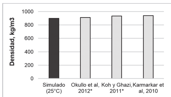
Figura 2. Densidad del aceite de J. curcas . *Okullo et al. , 2012 y Koh y Ghazi, 2011 reportan rangos, con valores mínimos de 907,36kg/m 3 y 860kg/m 3 , respectivamente.
