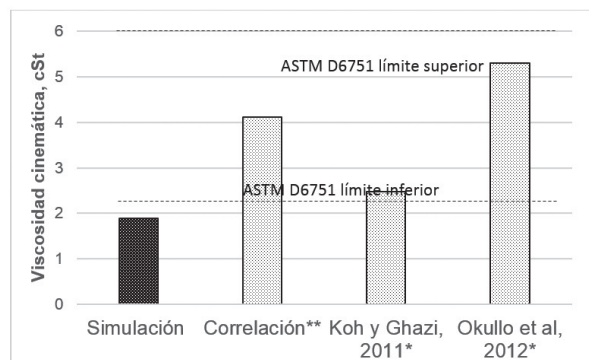
Figura 7. Viscosidad cinemática del biodiesel de J. curcas . * Koh y Ghazi, 2011 y Okullo et al. , 2012 reportan rangos, con valores mínimos de 2,23 5cSt, respectivamente. **Ramírez-Verduzco et al. , 2011.
