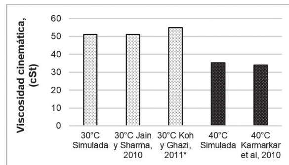
Figura 3. Viscosidad cinemática del aceite de J. curcas *Koh y Ghazi, 2011 reportan un rango, con valor mínimo de 37cSt.
