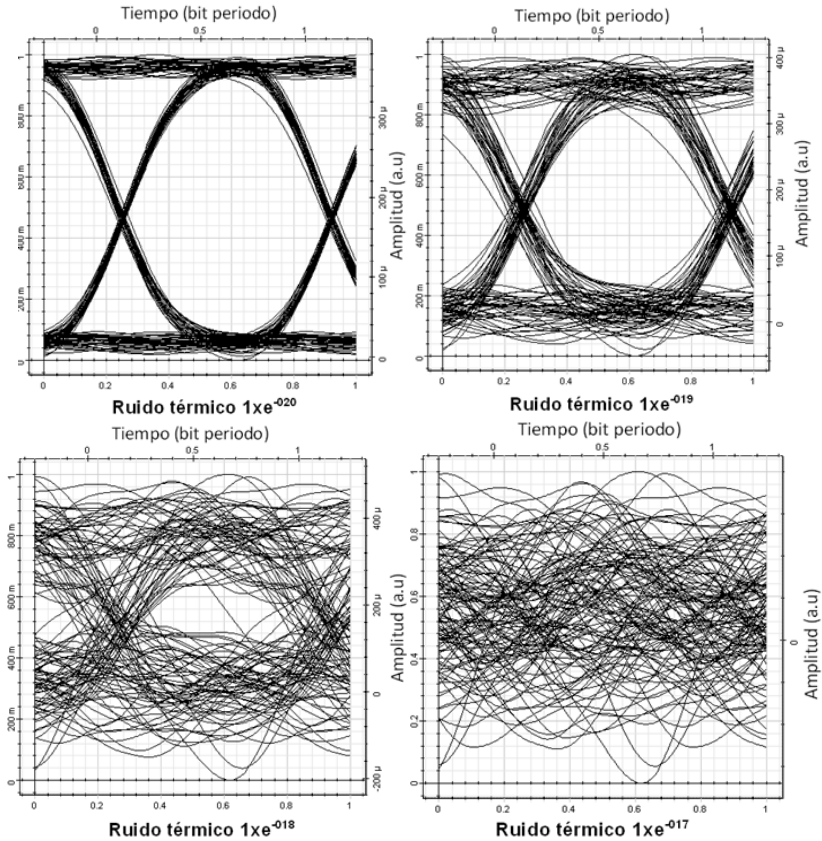
Fig. 4. Medida de diagramas de ojo para diferentes valores de ruido térmico medidos a la salida del DEMUX. Escala de tiempo 0,2 ns/div
