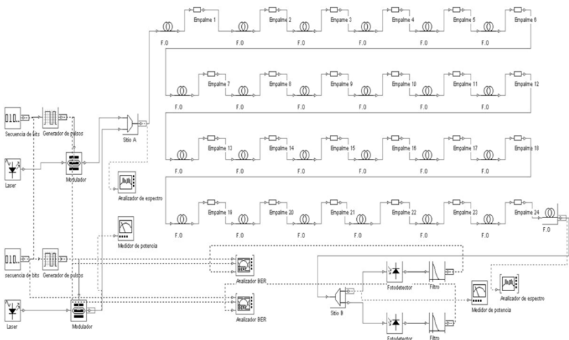
Fig. 2. Simulación Computacional en Optysistem V.7 (Versión evaluativa) del enlace de fibra óptica bajo una configuración SDH-WDM
