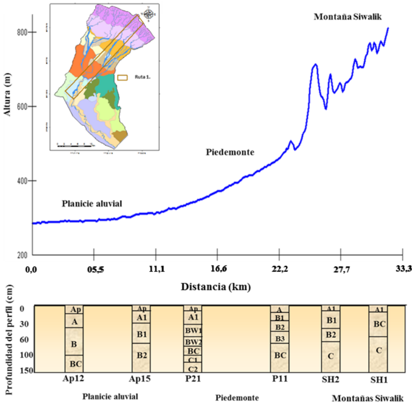
Figura 5. Descripción de las unidades fisiográficas de la cuenca Solani. Transecta 1
