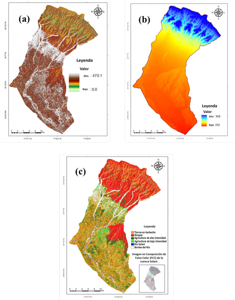
Figura 3. Procesamiento digital de imágenes (PDI) para el análisis fisiográfico de la cuenca Solani. (a) Análisis de Componentes Principales; (b) Modelo Digital de Elevación (MDE); (c) Transformación de la imagen-Clasificación supervisada
