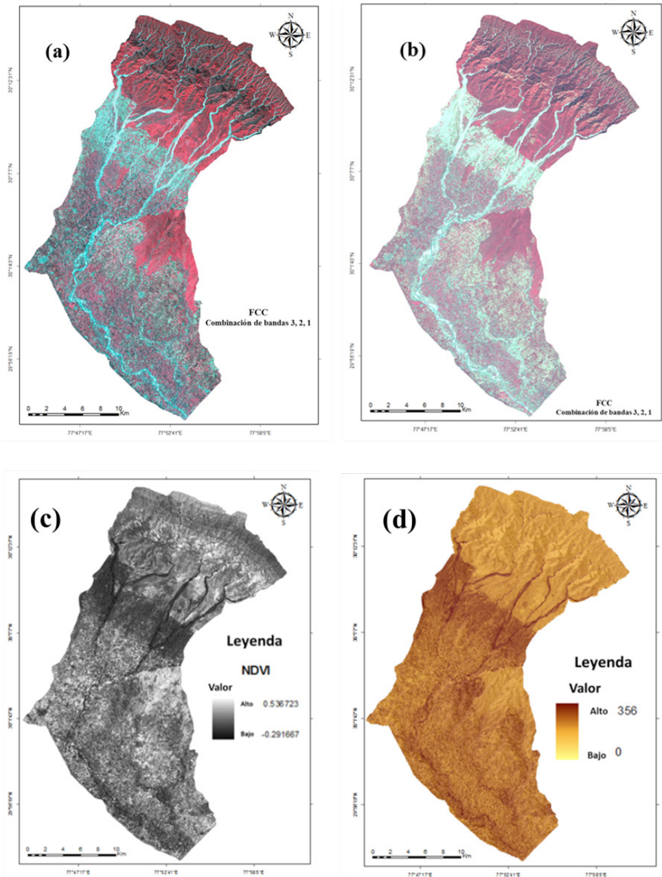
Figura 2. Procesamiento digital de imágenes (PDI) para el análisis fisiográfico de la cuenca Solani. Composición falso color de la imagen (a) LANDSAT TM (noviembre, 2000) y (b) IRS LISS III (octubre, 2005); (c) Relación de bandas (Band ratio) - NDVI; (d) Transformación de imagen - Índice de Brillantez del Suelo (SBI)
