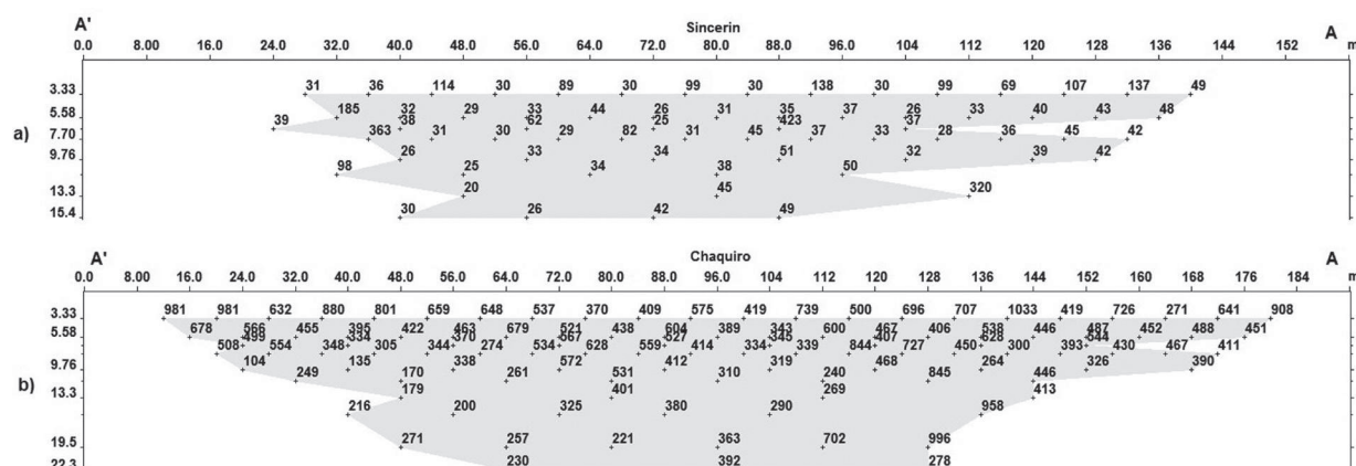
FIGURA 11. Pseudosecciones de resistividad aparente que muestran las coordenadas de los datos tomados bajo superficie con el ensayo dipolo-dipolo. a) Sincerín. b) El Chaquiro.
