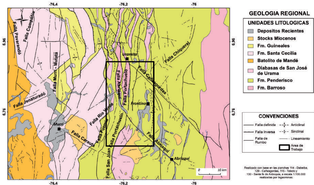
FIGURA 2. Geología regional del área de estudio. Modificado de Noriega y Caballero (2015).
