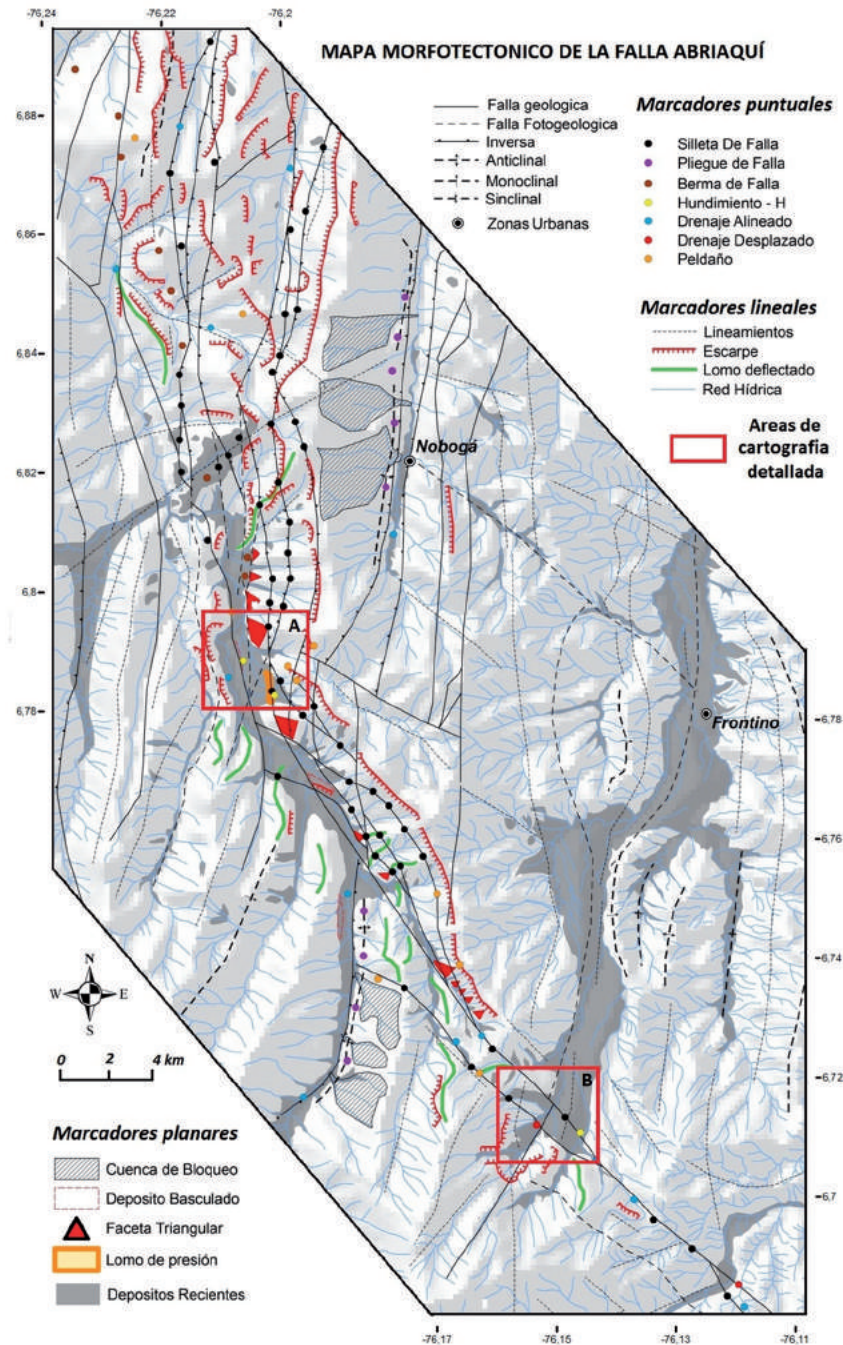
FIGURA 3. Mapa morfotectónico simplificado de la Falla Abriaquí y las áreas de cartografía detallada donde se realizó la exploración geofísica; las coordenadas se encuentran en grados decimales. a) Sincerín. b) El Chaquiro. Modificado de Noriega y Caballero (2015).
