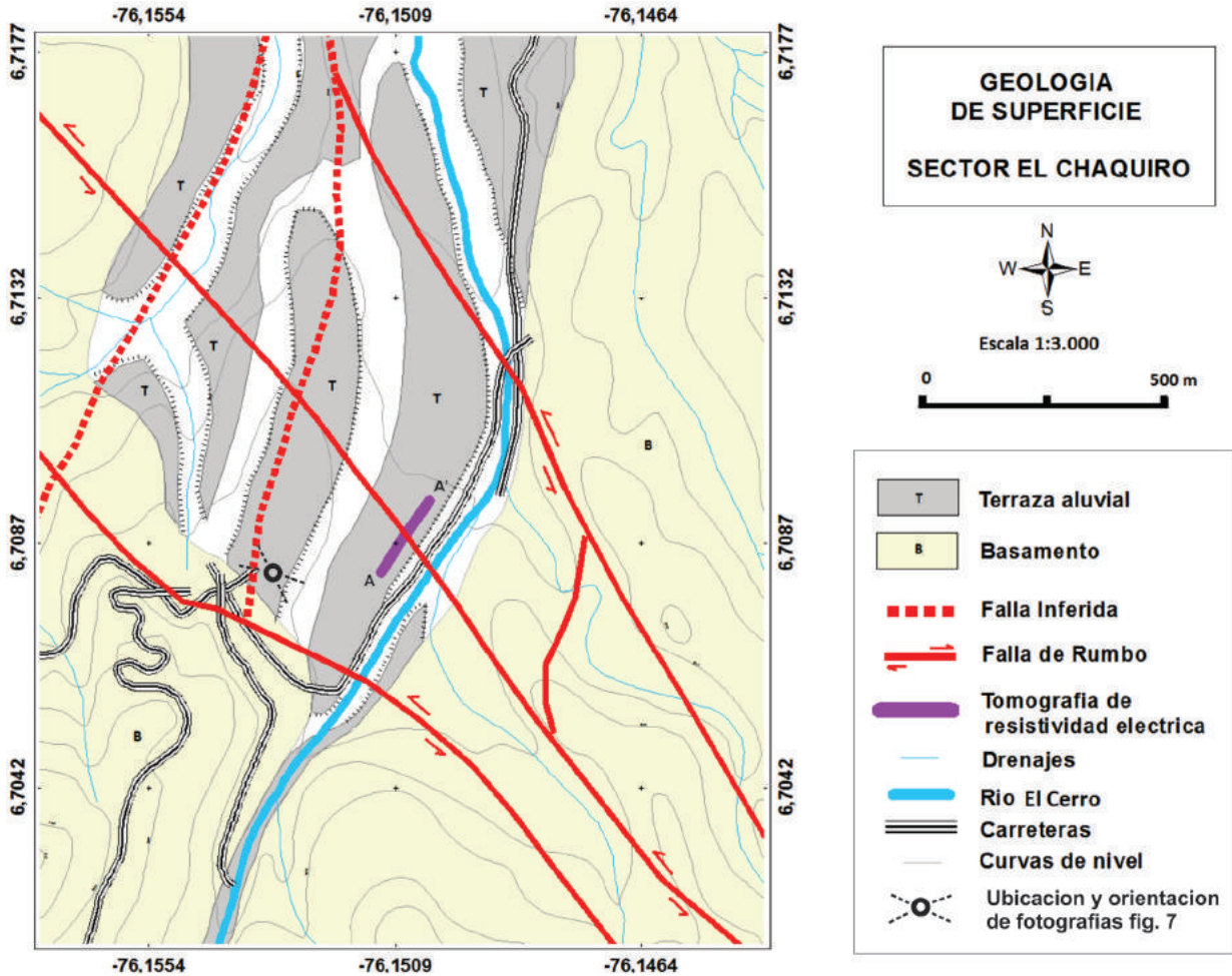
FIGURA 6. Geología de superficie en el sector del río El Cerro, localidad El Chaquiro, y ubicación del perfil de resistividad eléctrica. La ubicación de la figura dentro del área de estudio se encuentra en la FIGURA 3, recuadro b. Las coordenadas del mapa se encuentran en grados decimales.
