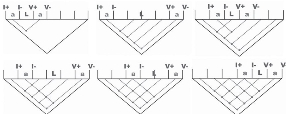
FIGURA 9. Representación de la elaboración de la pseudosección en el ensayo dipolo-dipolo. Los símbolos I^+ e I^- denotan la ubicación de los electrodos de corriente, y los símbolos V^+ y V^- hacen referencia a la ubicación de los electrodos de potencial. Esta representación corresponde al esquema de conmutación de electrodos implementado en este estudio, donde mediante arreglos de siete electrodos con diferentes separaciones se construyeron las pseudosecciones
