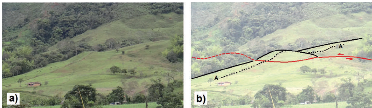
FIGURA 5. Lomo de presión sobre abanico aluvial en el sector de Sincerín. Tomada de Noriega y Caballero (2015). El perfil A-A' se señala en planta en la FIGURA 4.
