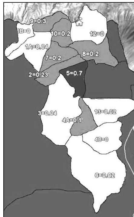
Figura 8. Distribución de las densidades de las tropillas de machos, \alpha=0.05 . Sector(n) = densidad (grupos/km 2 ).
