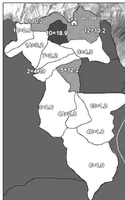
Figura 6. Distribución de las densidades de la población, \alpha=0.05 . Sector(n) = densidad (gua/km 2 ).
