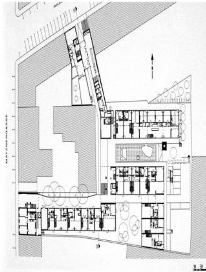
Figura 6- El equipo de proyecto propone una arquitectura de participación con el usuario y con las instituciones. Herederos de la amplia tradición vienesa de cooperativas de vivienda, que se remonta a los conocidos Höffe de la década del 20, su obra hace un especial hincapié en nuevos modos de vida colectiva, dotando a los grupos de vivienda de una serie de servicios que refuerzan el sentido de comunidad de los habitantes. La diversidad tipológica, en este caso, busca la inclusión social. Viviendas especiales para discapacitados, inmigrantes y niños de familias desestructuradas, con usos comunes, como: café, sala de conciertos, guardería, centro de seminarios, piscinas y sauna. BKK-3 Cooperativa de viviendas
