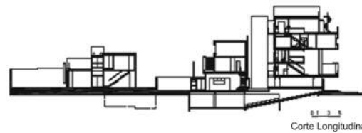
Figura 7- Es un conjunto de tres piezas edilicias de diferente altura y tipo de vivienda. El bloque frentista de la parcela es el más alto y acoge departamentos en dúplex, el segundo bloque está compuesto por tres viviendas en triplex y el tercero por dos viviendas en dos niveles. Provee distintos tipos de vivienda; en el segundo y tercer bloque se propone otorgarles carácter de vivienda individual, por lo que la mayor parte del espacio abierto no es común sino propio de las viviendas. Julián Berdichevsky – Joaquín Sánchez Gómez. Edificio Urbanverde, Cramer 1366, Ciudad de Buenos Aires, 2005. Summa+ 79 – 2006.
