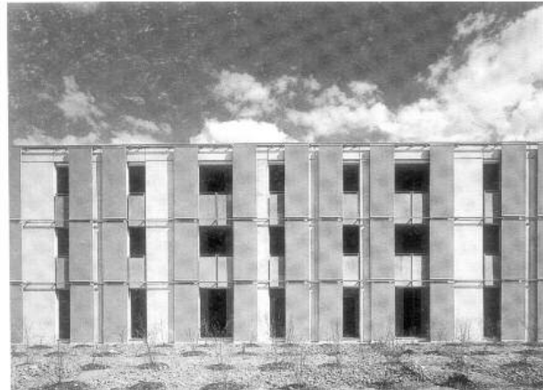
Figura 8- Sobre una estructura y paredes de hormigón armado, propone la envolvente y las particiones interiores con tecnología industrial, con elementos modulares y paneles móviles. Localiza los servicios, en una situación central permeable, y propone una serie de espacios similares situados en ambas caras del edificio, que se pueden usar de manera indistinta para estar, dormir o trabajar, relacionados con paneles móviles. Florian Riegler y Roger Riewe. 24 VIVIENDAS EN GRAZ, AUSTRIA. AV Monografías 56 – 1995.
