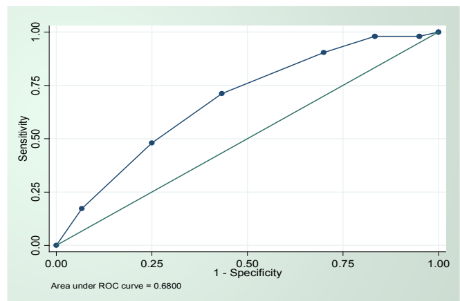
Figura 5. Curva ROC
