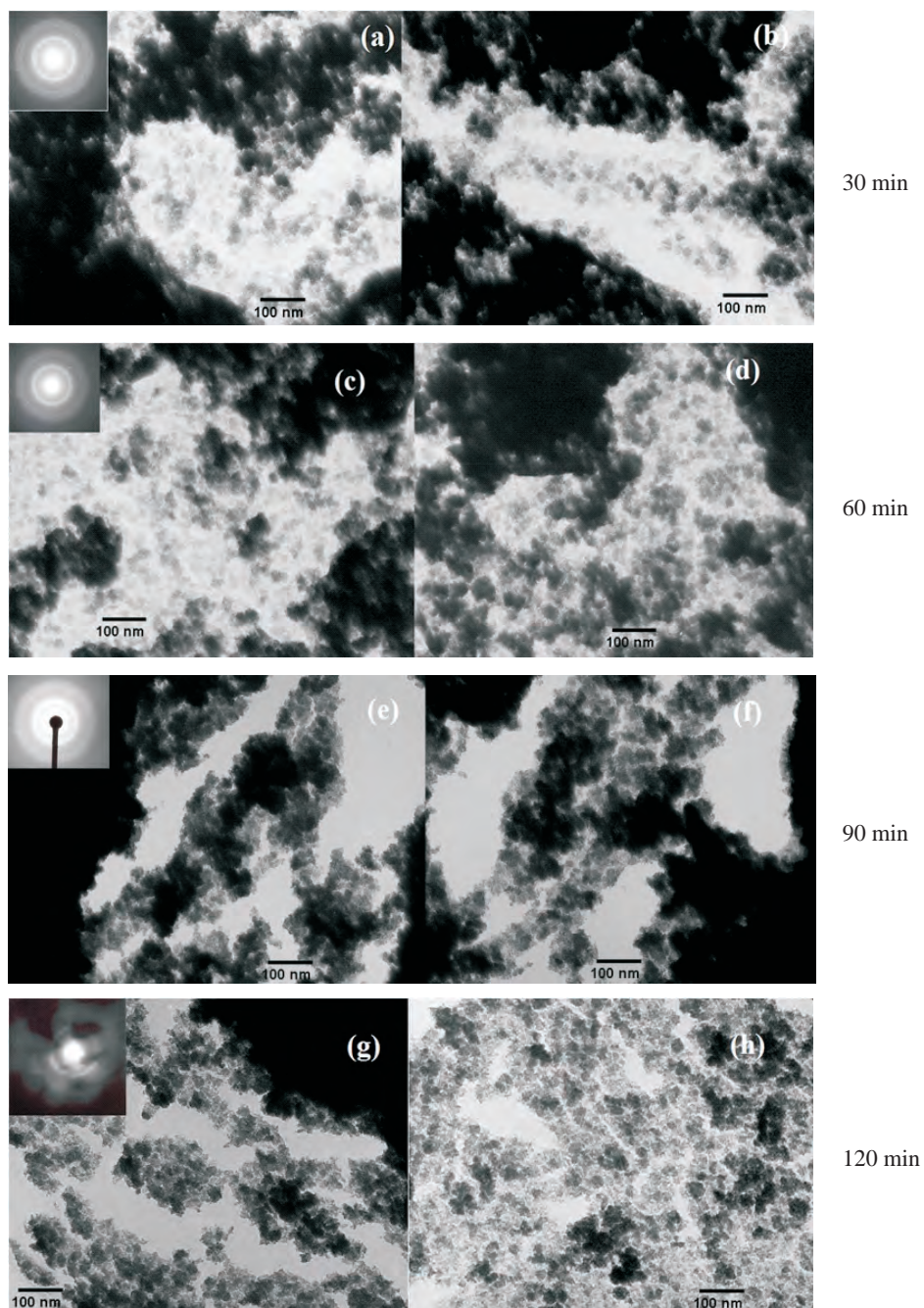
Figura 4. Micrografías electrónicas de transmisión para nanopartículas de \text{ZnO}_2 sintetizadas empleando los tiempos de sonicación indicados.
