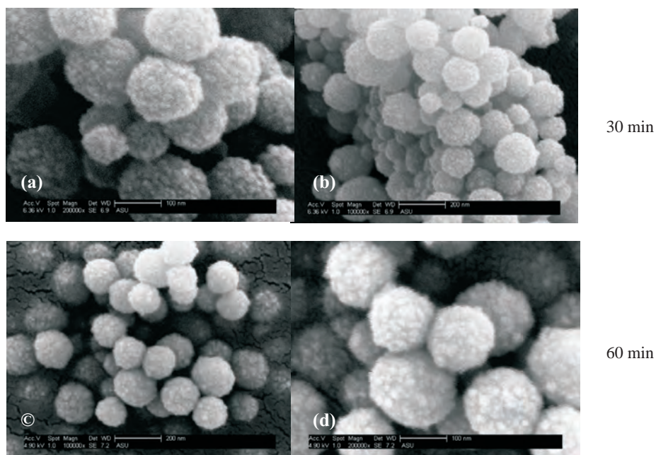
Figura 5. Micrografías electrónicas de barrido para nanopartículas obtenidas de coloides sonicados durante los tiempos indicados a 60^\circ\text{C} .
