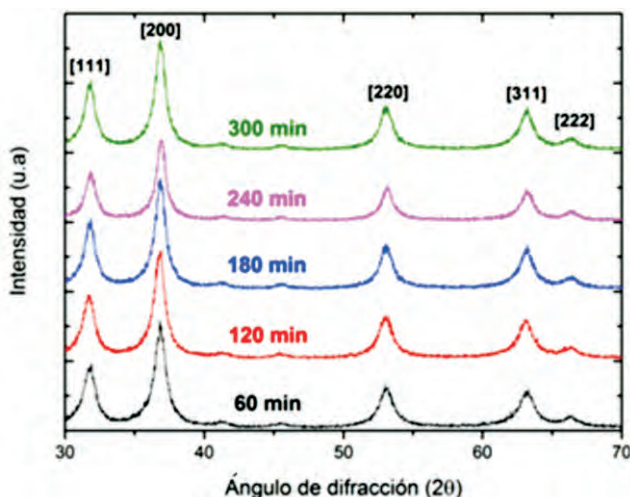
Figura 3. Difractograma de rayos X de nanopartículas de \text{ZnO}_2 sintetizadas para diferentes tiempos de sonicación
