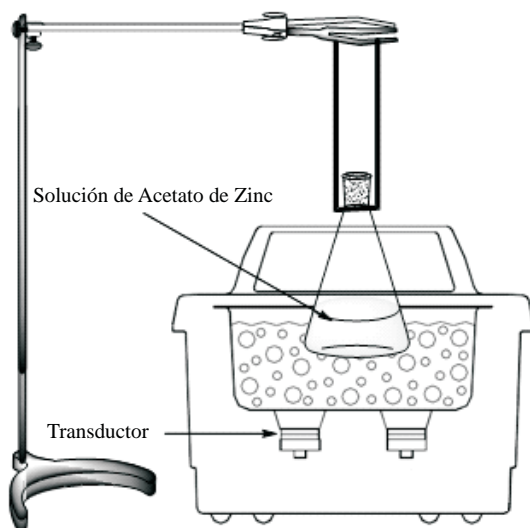
Figura 1. Montaje experimental empleado para la síntesis de nanopartículas de \text{ZnO}_2 usando ultrasonido.
