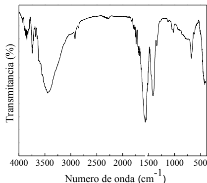
Figura 4. Espectros de infrarrojo con transformada de Fourier de nanopartículas \text{ZnO}_2 .
