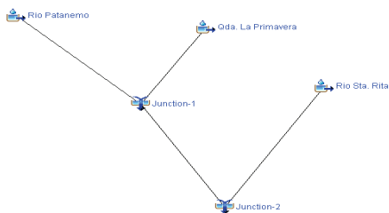
Figura 3: Modelo de la cuenca del río Patanemo (HEC – HMS)
