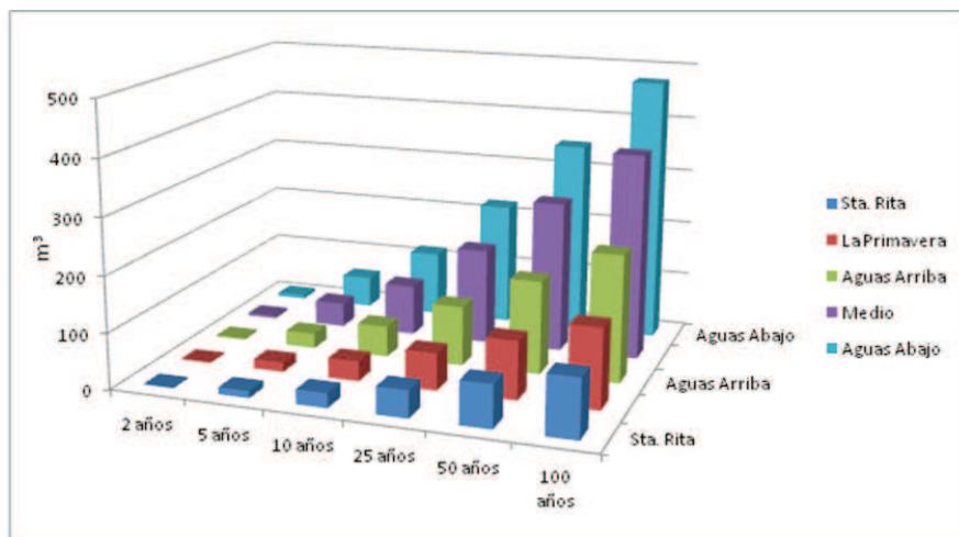
Gráfico 3. Caudales pico, cuenca del río Patanemo para diferentes periodos de retorno
