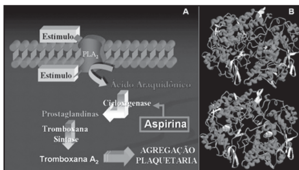
Figura 4 – A aspirina e seu mecanismo. A: produção de ácido araquidônico e tromboxano A 2 via metabólica-alvo da aspirina; B: enzima ciclooxigenase ligada ao ácido araquidônico (acima) e à aspirina (abaixo)
