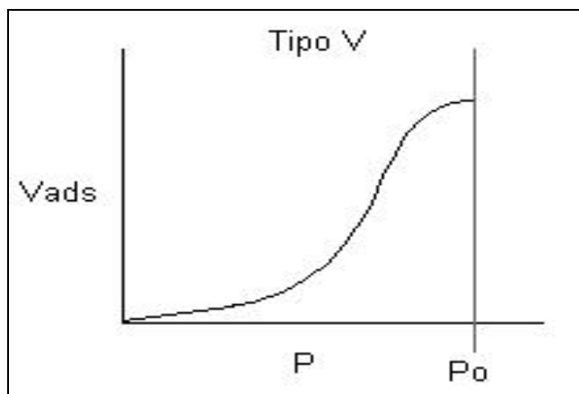
Figura 10. Isoterma de BET (Tipo V).
