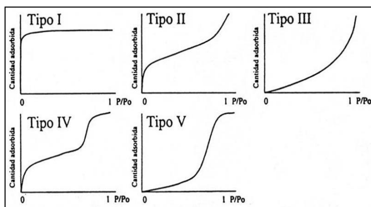
Figura 5. Tipos de isothermas.
