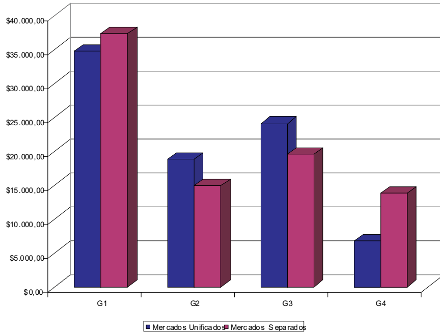
Figura 7. Ingresos totales de cada generador para cada mercado
