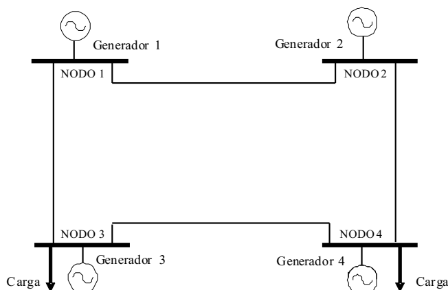
Figura 4. Sistema de prueba de cuatro nodos
