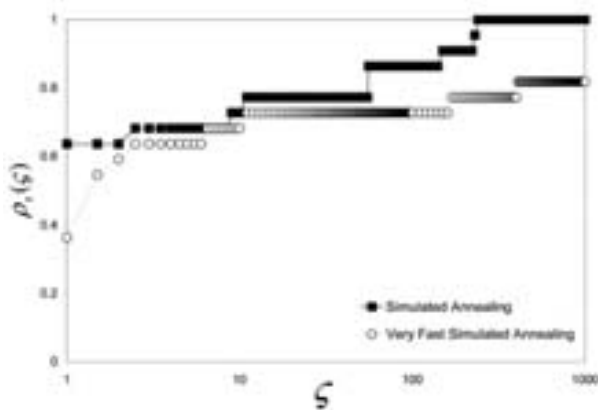
Figura 3. Perfiles de comportamiento numérico para la métrica t_{p,s}^d = \frac{\hat{f}_{obj} - f_{obj}^*}{f_{obj}^{iv} - f_{obj}^*} empleando los métodos estocásticos SA y VFSA en cálculos termodinámicos
