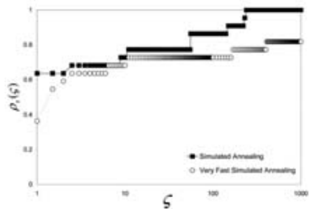
Figura 4. Perfiles de comportamiento numérico para la métrica t_{p,s}^{NFE} = N\hat{F}E empleando los métodos estocásticos SA y VFSA en cálculos termodinámicos
