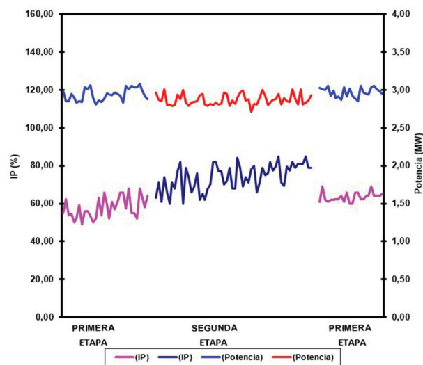
Figura 3. Comportamiento del índice de preparación de la caña en la potencia demandada del tándem
