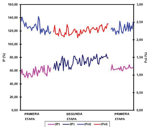
Figura 1. Comportamiento del índice de preparación de la caña sobre el % Pol en bagazo final
