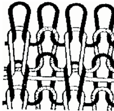
Figura 3. Estructura milano: dos secciones simples de fibras tejidas en dos juegos separados de agujas (trama 2 y 3), los cuales están sujetos por una hilera 1x1 (trama 1)
