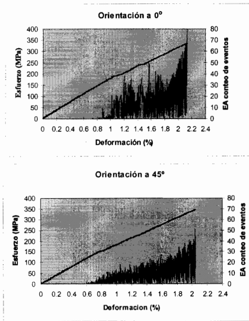
Figura 6. Curvas de esfuerzo-deformación-EA de probetas a: a) 0°, b) 45° y c) 90° (continúa ...)
