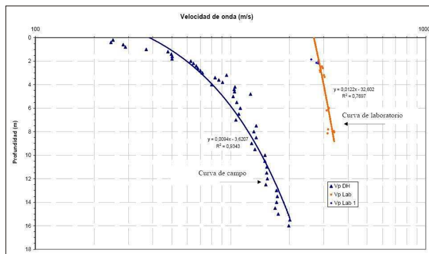
Figura 2. Variación de las velocidades de ondas, V_p , con la profundidad, para campo y laboratorio, respectivamente
