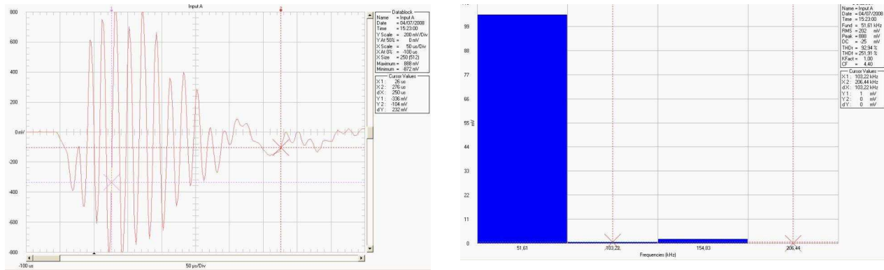
Figura 1. Oscilograma de laboratorio para una muestra de roca lodosa de la Cordillera Oriental y su espectro de frecuencias, obtenido mediante el osciloscopio Fluke® de la Universidad Nacional, Bogotá (2008) en [19]
