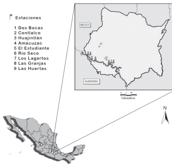
Figura 1. Localización de las estaciones de colecta en el Río Amacuzac, Morelos, México. (Elaborado por Abigail Barrientos, 2008) (Tomado de Távira, 2010).
