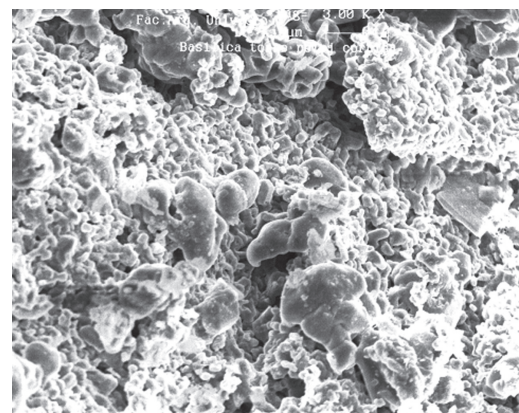
Figura 4: Micrografía de SEM a X3,000. Piedra rosa sin consolidar. Piedra rosa de la torre del reloj de la Basílica Colegiata de Nuestra Señora de Guanajuato en Guanajuato, Gto., México.
