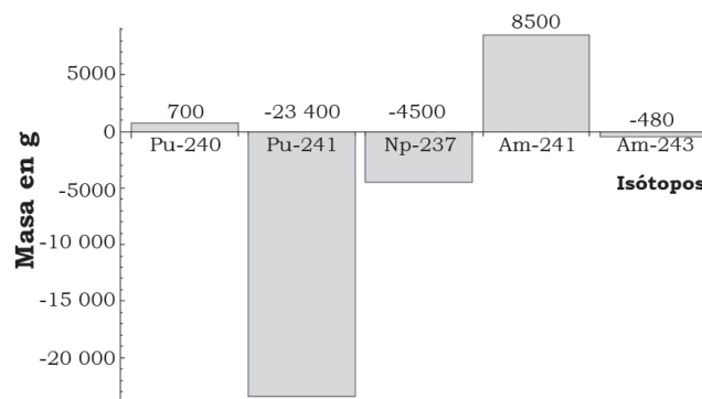
Figura 9. Inventario de masas para el total del tiempo de irradiación.
