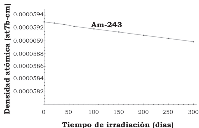
Figura 8. Evolución de la densidad atómica del ^{243}\text{Am} en función del tiempo de irradiación.
