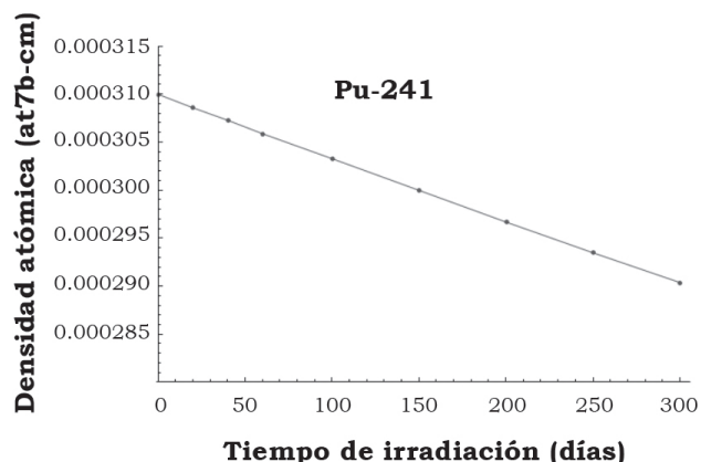
Figura 5. Evolución de la densidad atómica del ^{241}\text{Pu} en función del tiempo de irradiación.
