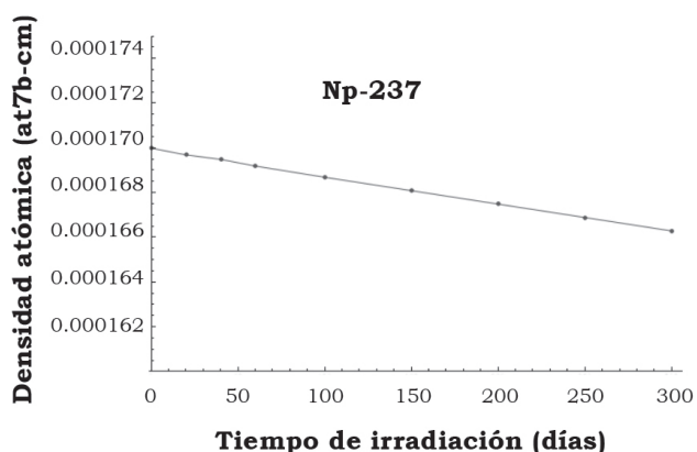
Figura 6. Evolución de la densidad atómica del ^{237}\text{Np} en función del tiempo de irradiación.
