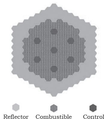
Figura 1. Configuración para la disposición radial del núcleo del reactor. Fuente: Martín et al. (2011).
