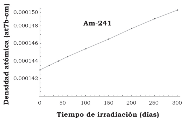
Figura 7. Evolución de la densidad atómica del ^{241}\text{Am} en función del tiempo de irradiación.
