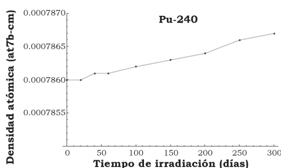
Figura 4. Evolución de la densidad atómica del 240 Pu en función del tiempo de irradiación. Fuente: Elaboración propia.
