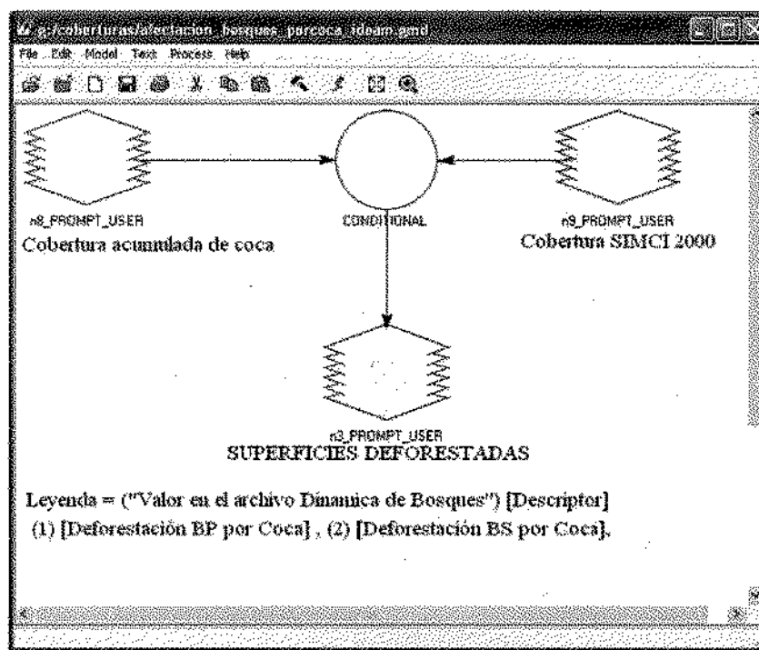
Figura 14. Modelo condicional
