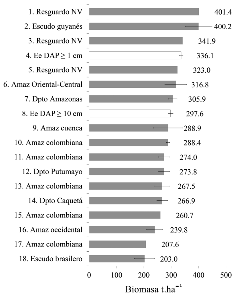
Figura 3. Comparación de la biomasa ( t.ha^{-1} ) estimada en este estudio (Ee) para árboles con DAP \geq 1 cm y DAP \geq 10 cm, con otros reportes para el medio Caquetá, la Amazonia colombiana y la cuenca Amazónica. Se presentan los valores reportados por los diferentes autores, y su respectiva desviación estándar cuando esta estuvo disponible. Fuente: Álvarez et al. (2017) (13); Anaya et al. (2009) (15); Asner et al. (2012) (17); Baccini et al. (2012) (5); Galindo et al. (2011) (7, 11, 12, 14); Londoño (2011) (3); Mitchard et al. (2014) (2, 6, 9, 16, 18); Phillips et al. (2016) (10); Saatchi et al. (2011) (1).
