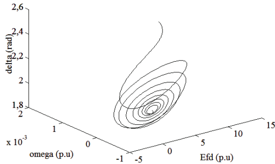
Figura 17 Región 5 (Pt=2,08 y D=220)
