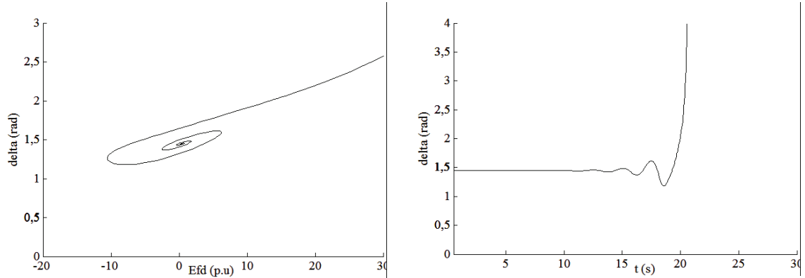
Figura 23 Divergencia para el punto de equilibrio correspondiente a Pt=1,8 y D=70
