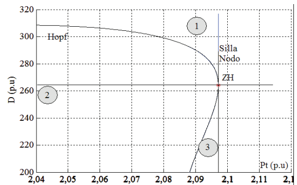
Figura 24 a) Diagrama de bifurcaciones para puntos ZH con s=-1 y \theta < 0 [10]. b) Definición de regiones en cercanías del punto Zero-Hopf
