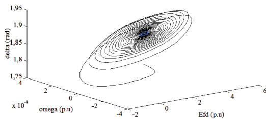
Figura 25 Región 1 (Pt=2,09 y D=310). La trayectoria converge a un punto de equilibrio estable
