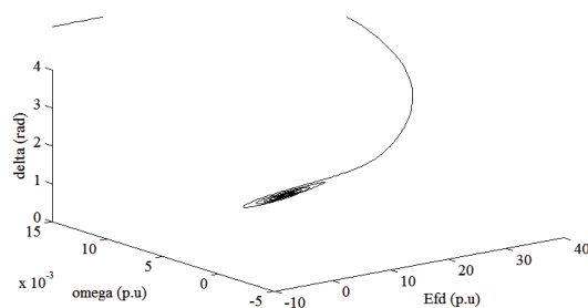
Figura 26 Región 2 (Pt=2,04 y D=260). Zona de inestabilidad
