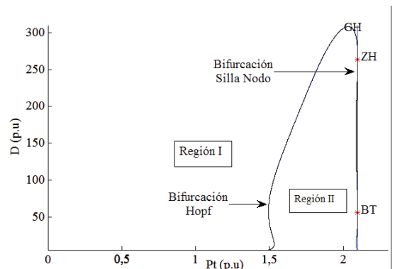
Figura 19 Diagrama de bifurcaciones 2 dimensional para el SMIB con limitador
