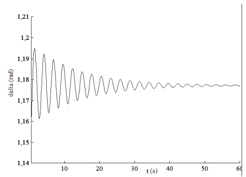
Figura 22 Convergencia para el punto de equilibrio correspondiente a P_t=1,5 y D=150
