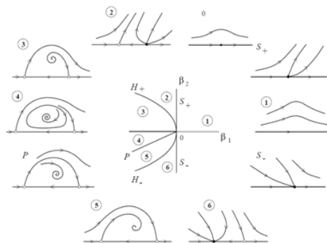
Figura 11 Diagrama de bifurcaciones de la forma normal truncada, para ZH, con s=1 y \theta < 0 [10]
