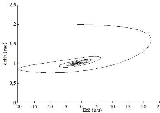
Figura 20 Convergencia para el punto de equilibrio correspondiente a P_t=1,3 y D=110
