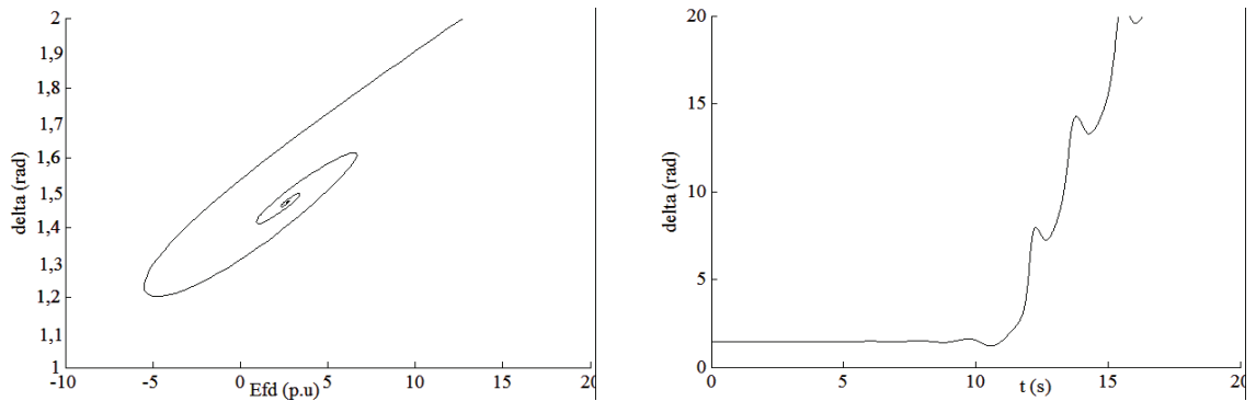
Figura 9 Divergencia para P_t=1,8 y D=70 . a) Retrato de fase b) Respuesta en el tiempo
