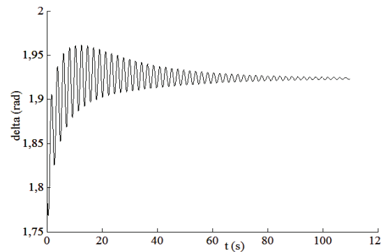
Figura 13 Región 1 ( P_t=2,08 y D=300 ). La trayectoria converge a un punto de equilibrio estable
