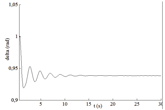
Figura 21 Convergencia para el punto de equilibrio correspondiente a P_t=1,2 y D=40
