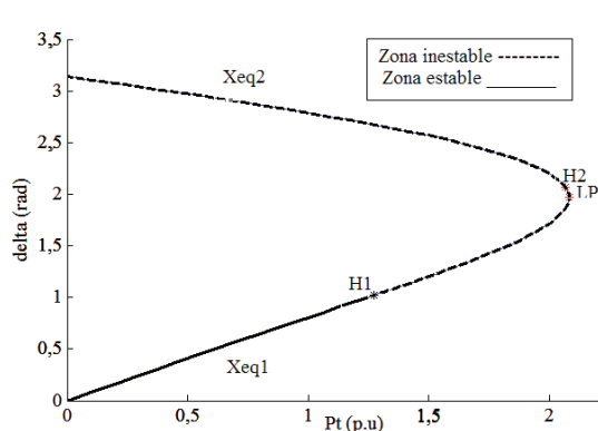
Figura 3 Diagrama de bifurcaciones para la variable \delta con D=110
