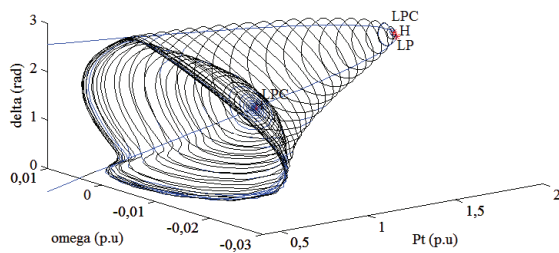
Figura 4 Disminución del ciclo límite inestable y colisión con punto estable en H^1
