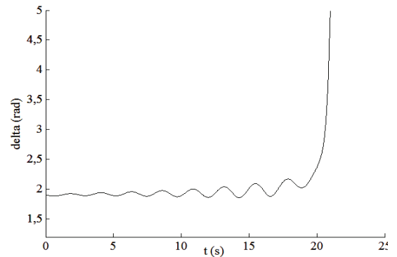
Figura 15 Región 3 (Pt=2,04 y D=260). Aparición de una órbita cuasiperiódica (o toro)
