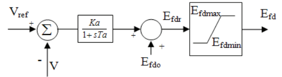
Figura 2 Sistema de excitación simplificado
