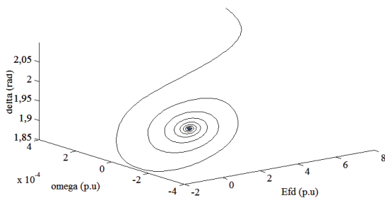
Figura 27 Región 3 (Pt=2,092 y D=220). Zona de inestabilidad
