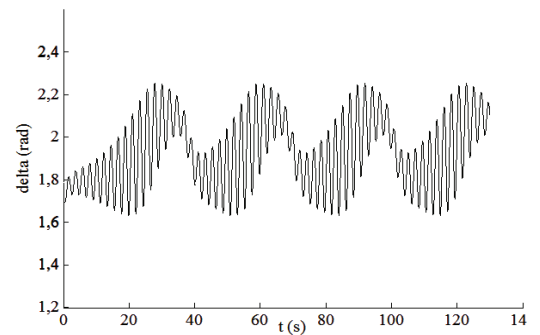
Figura 15 Región 3 (Pt=2,04 y D=260). Aparición de una órbita cuasiperiódica (o toro)
