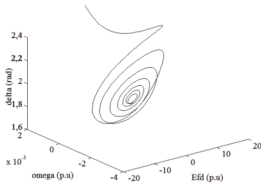
Figura 16 Región 4 (Pt=2,06 y D=220)
