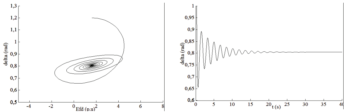
Figura 8 Convergencia para el punto P_t=1 y D=50 . a) Retrato de fase b) Respuesta en el tiempo
