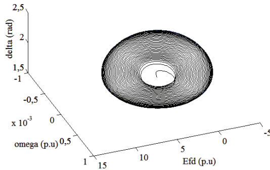
Figura 14 Región 2 (Pt=2,07 y D=280). Influencia de un ciclo límite
