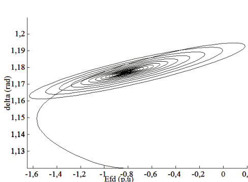
Figura 22 Convergencia para el punto de equilibrio correspondiente a P_t=1,5 y D=150
