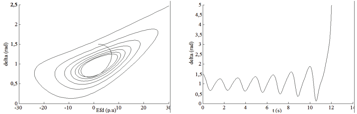
Figura 6 Divergencia para el punto P_t=1,2 y D=40 . a) Retrato de fase b) Respuesta en el tiempo
