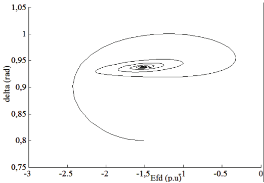
Figura 21 Convergencia para el punto de equilibrio correspondiente a P_t=1,2 y D=40
