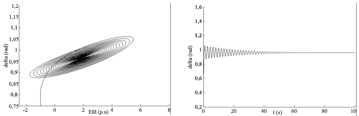
Figura 7 Convergencia para P_t=1,2 y D=100 . a) Retrato de fase b) Respuesta en el tiempo
