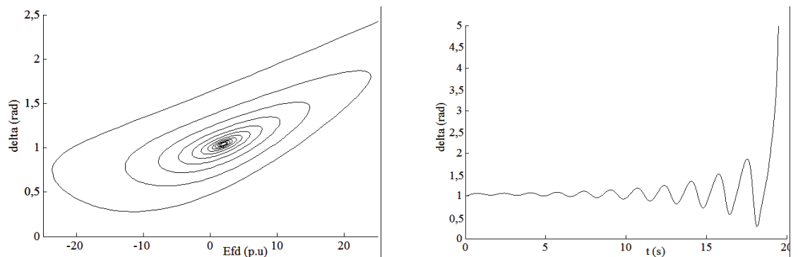
Figura 10 Divergencia para P_t=1,3 y D=50 . a) Retrato de fase b) Respuesta en el tiempo
