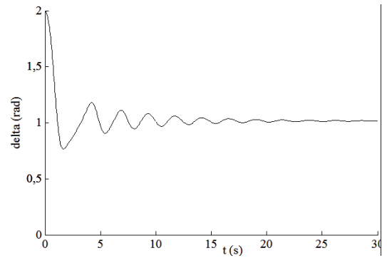
Figura 20 Convergencia para el punto de equilibrio correspondiente a P_t=1,3 y D=110
