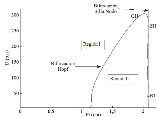
Figura 5 Diagrama de bifurcaciones 2-dimensional
