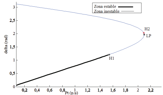
Figura 18 Diagrama de bifurcaciones uno dimensional para SMIB con limitador y D=110
