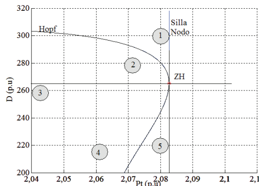
Figura 12 Análisis de estabilidad en las cercanías del punto Zero-Hopf ZH
