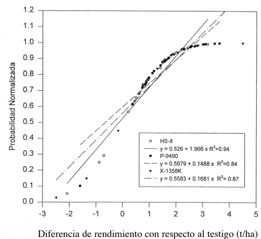
Figura 1. Relación de la confiabilidad con las diferencias de rendimiento de tres híbridos de maíz evaluados en Panamá.
