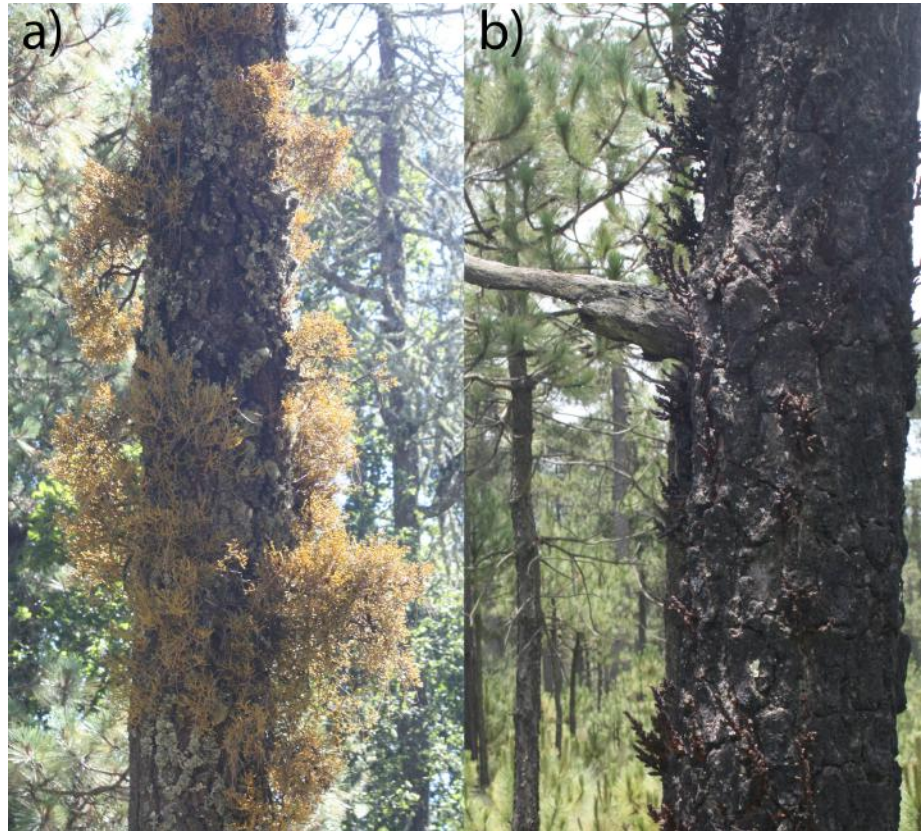
a) A. globosum y b) A. vaginatum parasitando el tronco de árboles de Pinus hartwegii . Figure 2. a) A. globosum and b) A. vaginatum parasitizing the stem of Pinus hartwegii trees.
