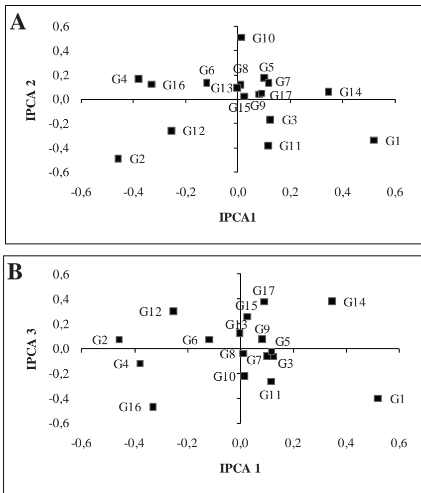
Figura 1. Gráficos biplots de modelo AMMI para dados de produtividade de grãos ( \text{kg ha}^{-1} ) de 17 linhagens de feijão (G1, LP 04-03; G2, LP 04-72; G3, CNFC 10408; G4, CNFC 10429; G5, BRS Valente; G6, Guapo Brilhante; G7, CHC 97-29; G8, CHP 98-59; G9, GEN C 2-1-1; G10, GEN C 2-1-3; G11, Pérola; G12, Carioca; G13, SM 0707; G14, SM 1007; G15, SM 1207; G16, TB 02-20; e G17, TB 02-21) avaliadas em 10 ambientes durante o biênio 2008 e 2009, A: biplot AMMI 2 – primeiro componente principal (IPCA 1) x segundo componente principal (IPCA 2); B: biplot AMMI 3 – primeiro componente principal (IPCA 1) x terceiro componente principal (IPCA 3).
